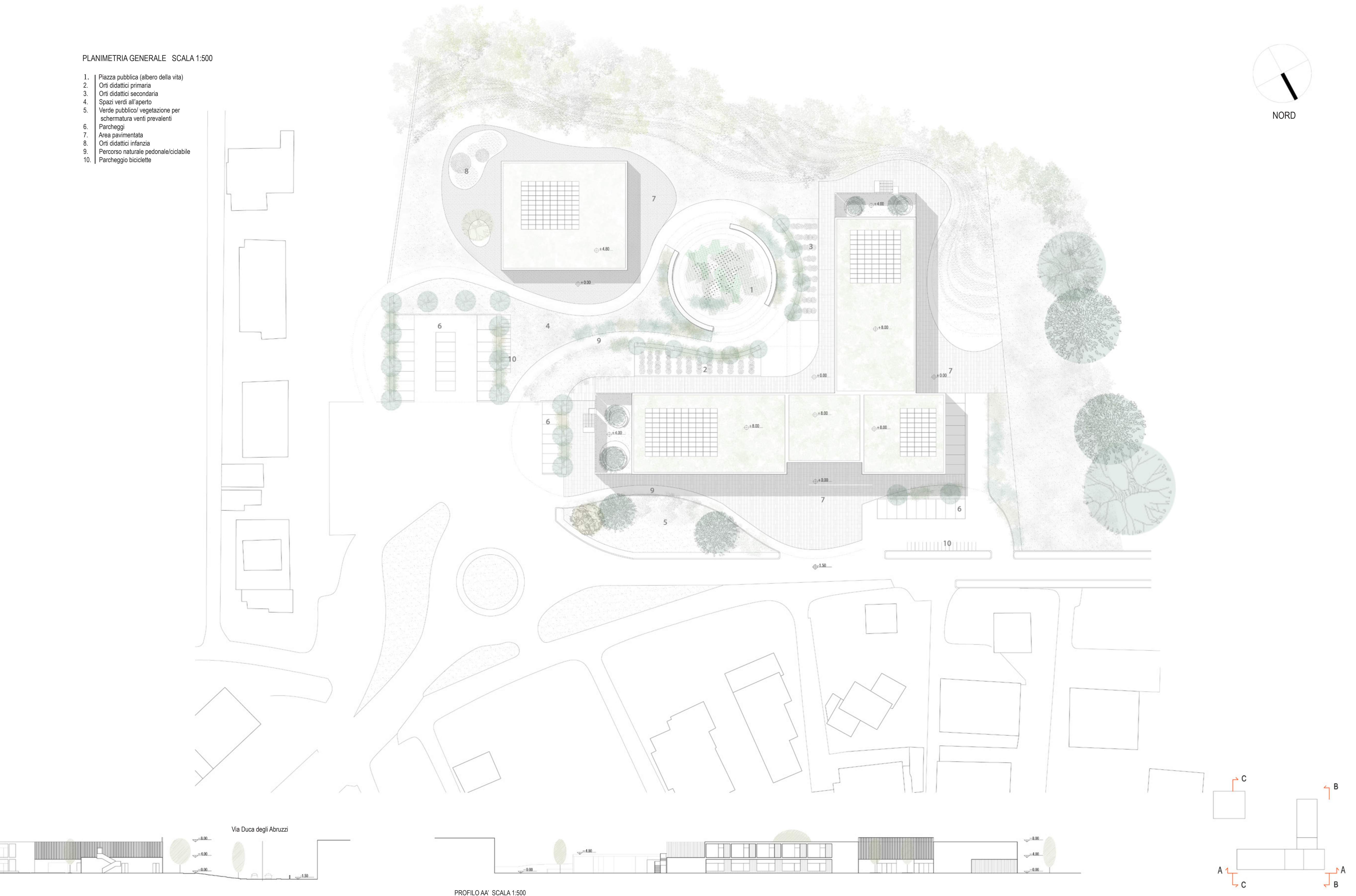
PROFILO AA' SCALA 1:500
